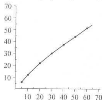
Рис. 29. Результаты тарировки 3 электролитических датчиков дыхания для исследования естественного и исполнительского дыхания методом электропневмографии
