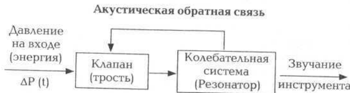
Рис. 2. Структурная схема автоколебательной системы духовых инструментов
